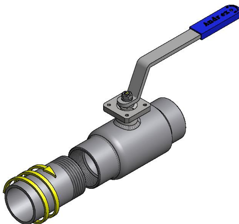
Rys. 8 Montaż zaworu gwintowanego zewnątrz
