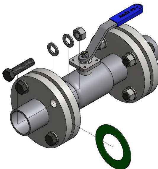
Rys. 5 Montaż zaworu kołnierzowego za pomocą śrub sześciokątnych
