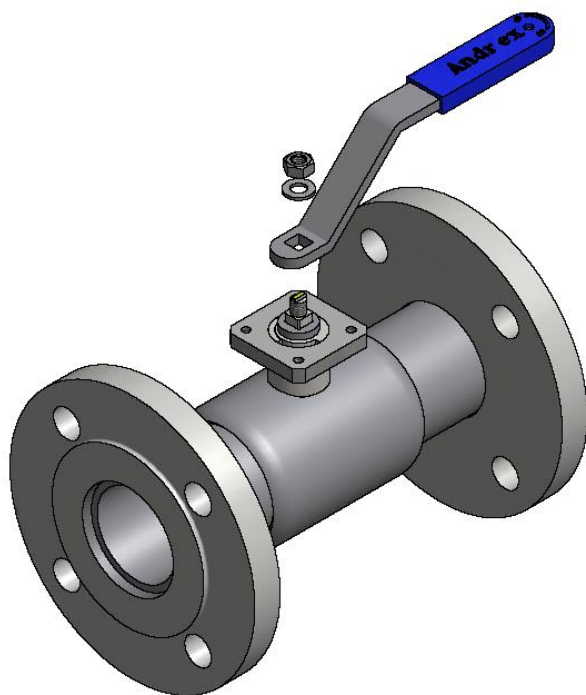
Rys. 13 Demontaż dźwigni sterującej.
