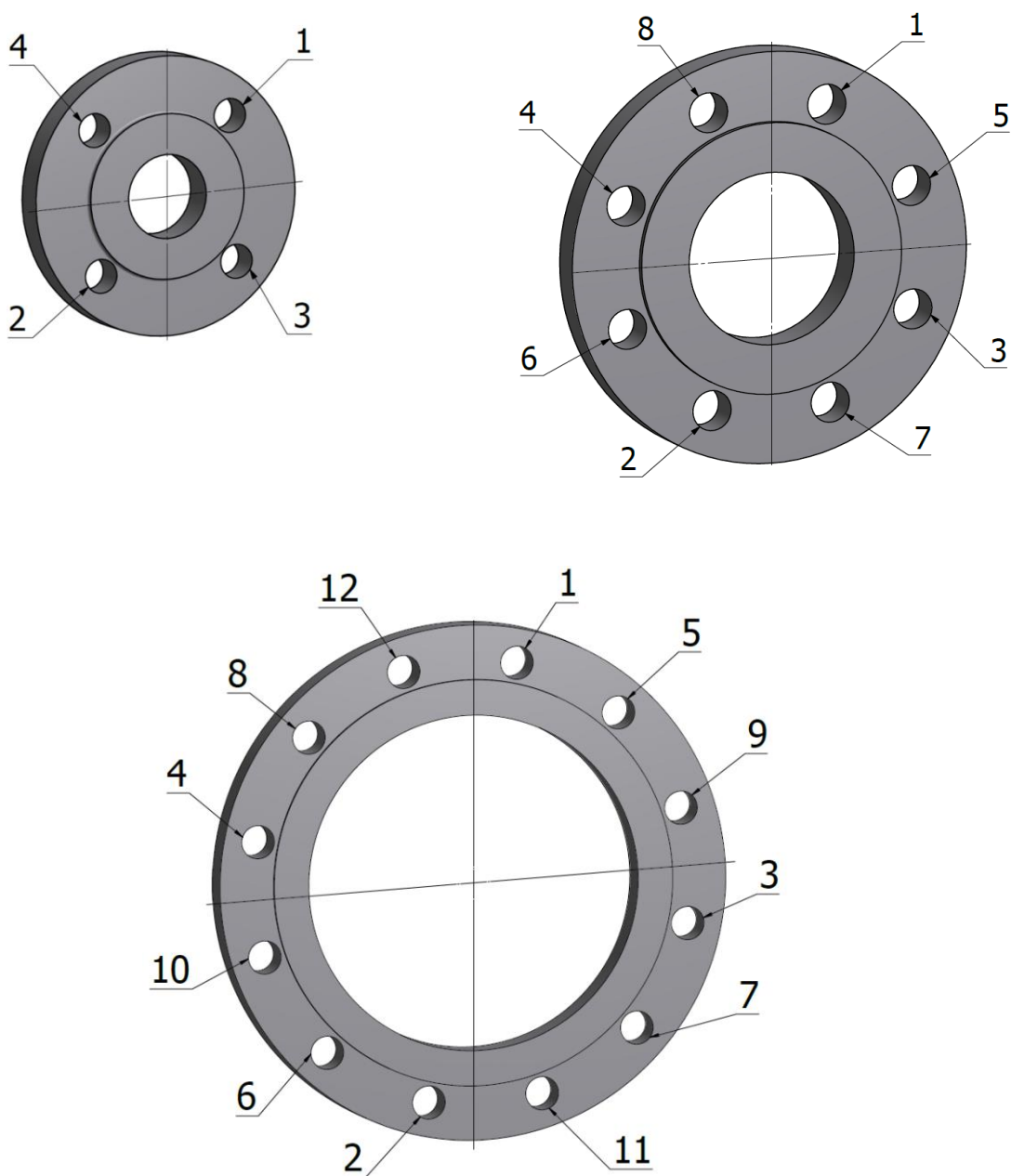
Rys. 4 Kolejność dokręcania śrub w kołnierzach
