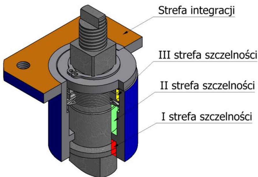
Rys. 9 Budowa dławnicy.
