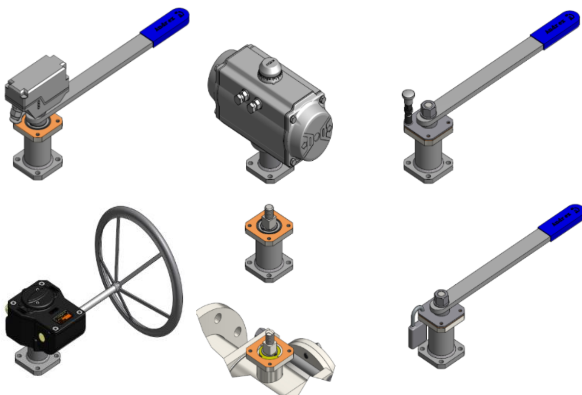
Rys. 15 Przykładowe rozwiązania sterujące armaturą.
