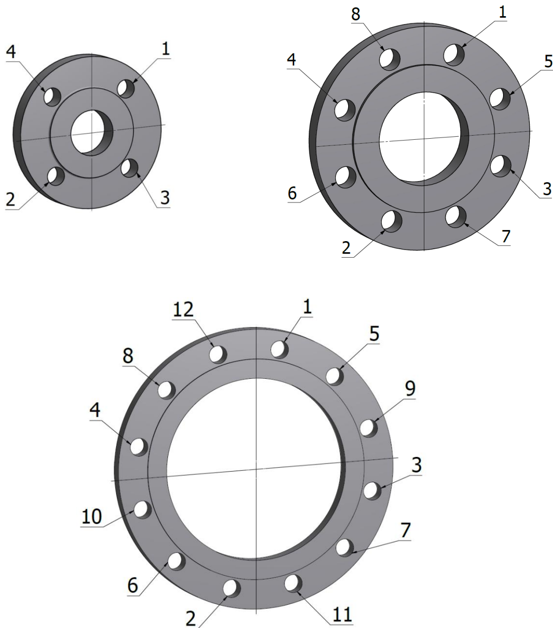
Rys. 4 Kolejność dokręcania śrub w kołnierzach
