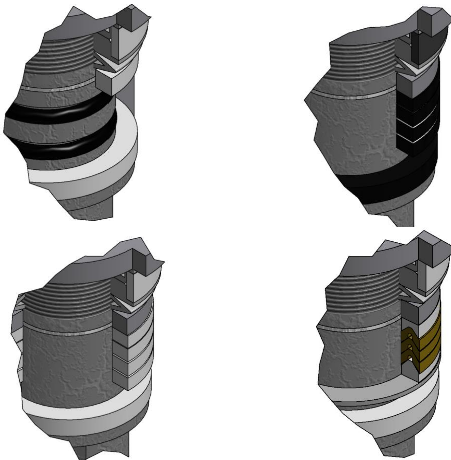
Rys. 10 Przykładowe wymienne uszczelnienie w dławnicy.
