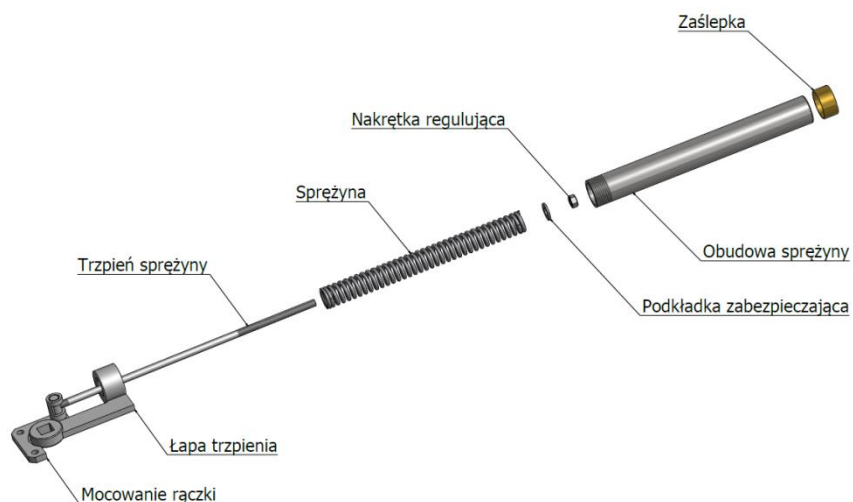
Rys. 16 Budowa rączki ze sprężyną powrotną.
