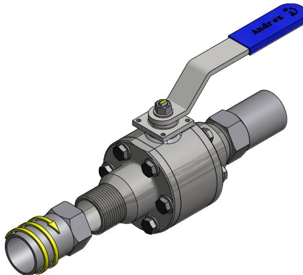
Rys. 7 Montaż zaworu gwintowanego zewnętrznie
