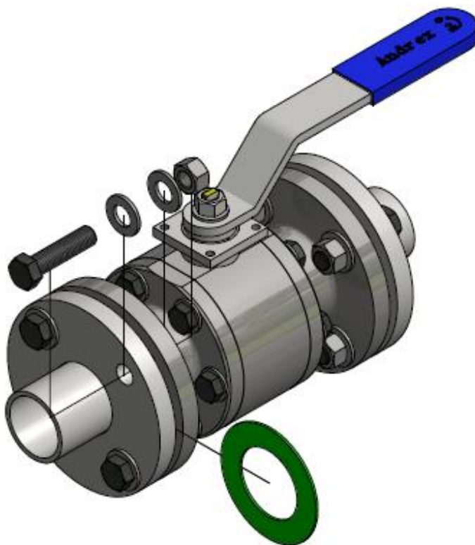
Rys. 5 Montaż zaworu kołnierzowego za pomocą śrub sześciokątnych
