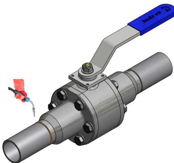
Rys. 6 Montaż zaworu do spawania
