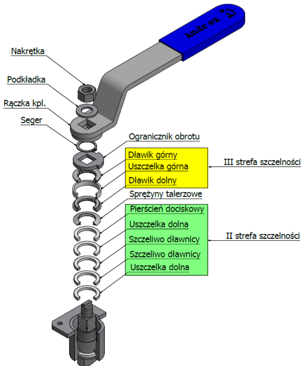
Rys. 11 Demontaż uszczelnienia w dławnicy.
